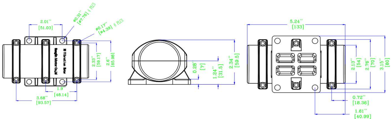
外形尺寸 Dimensions(Unit:Millimeter)
